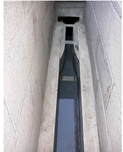
Venturi-flume in polyester of RVS Met / zonder laterale meetkamer
